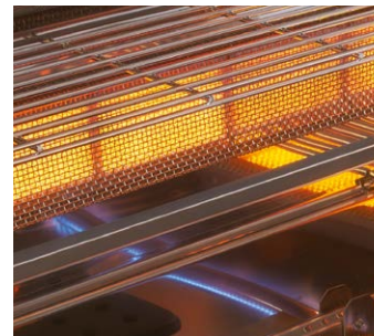
Keramisk infraröd bakre brännare
