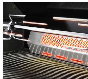
Infraröd bakre brännare för rotisseri
